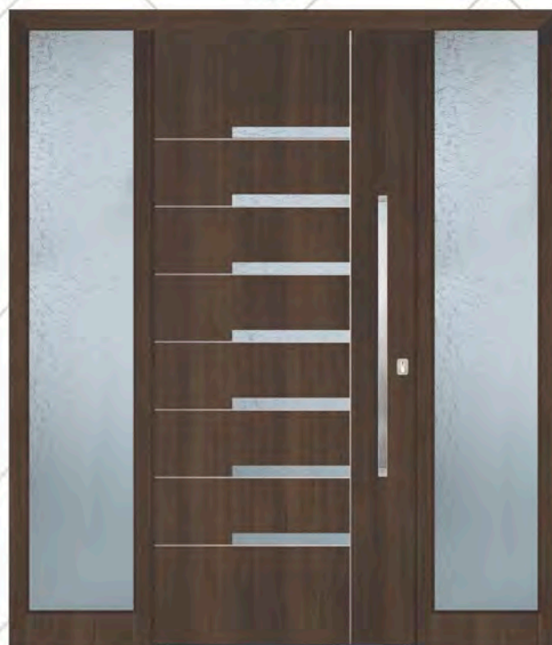
Model SOFIA Drvni dekor ORAH TAMNI FS Staklo MADRAS UADI Intarzije ČEŠLIANE Rukohvat KCR 950h Rozeta RKP 50 Dosvjetlo lijevo i desno MADRAS UADI
