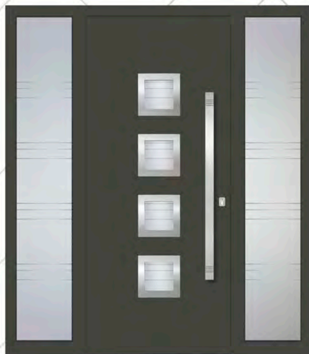
Model WARSZAWA RAL boja 7022 Staklo DPL Aplikacije POLIRANE Rukohvat DOK 115h Rozeta RKP 50 Dosljetlo lijevo i desno DPL
