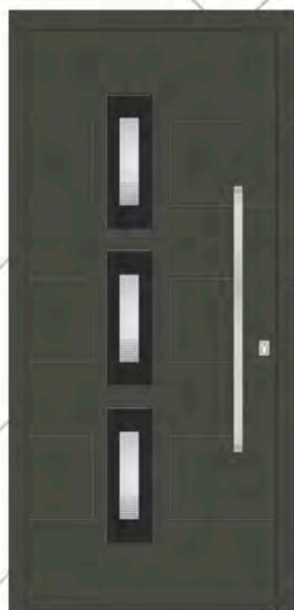
Modell/ Model MONACO Farbe RAL/ Ral colour 6015 Verglasung/ Glass DPZ Applikation Float Sicherheitsglas/ emailliert RAL 9005/ Application Float 6mm tempered enamelled RAL 9005 Griff/ Handle KPR 950h Rosette RKP 50
