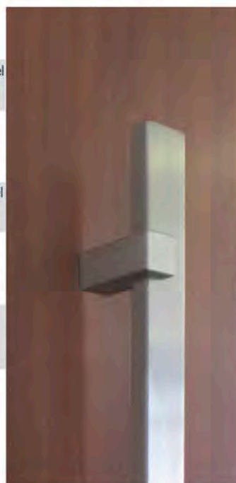
Griff KPD - Edelstahl poliert Breite 35mm, Stärke 20mm, Höhe 750mm KPD 750
